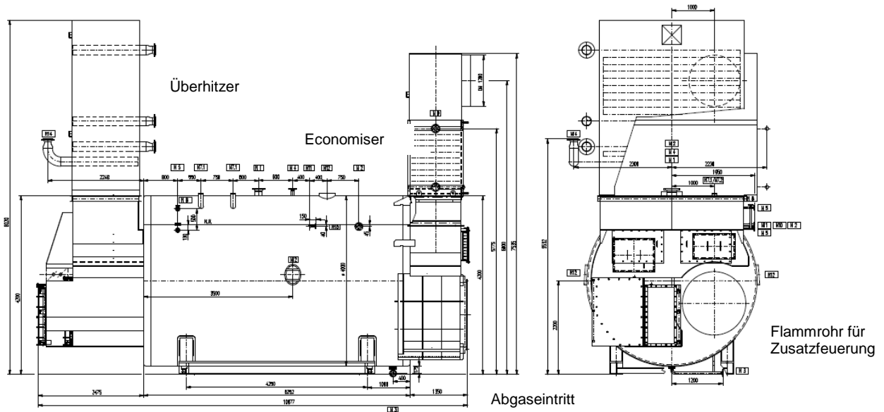
Bild 3 Kessel-Zusammenstellung
