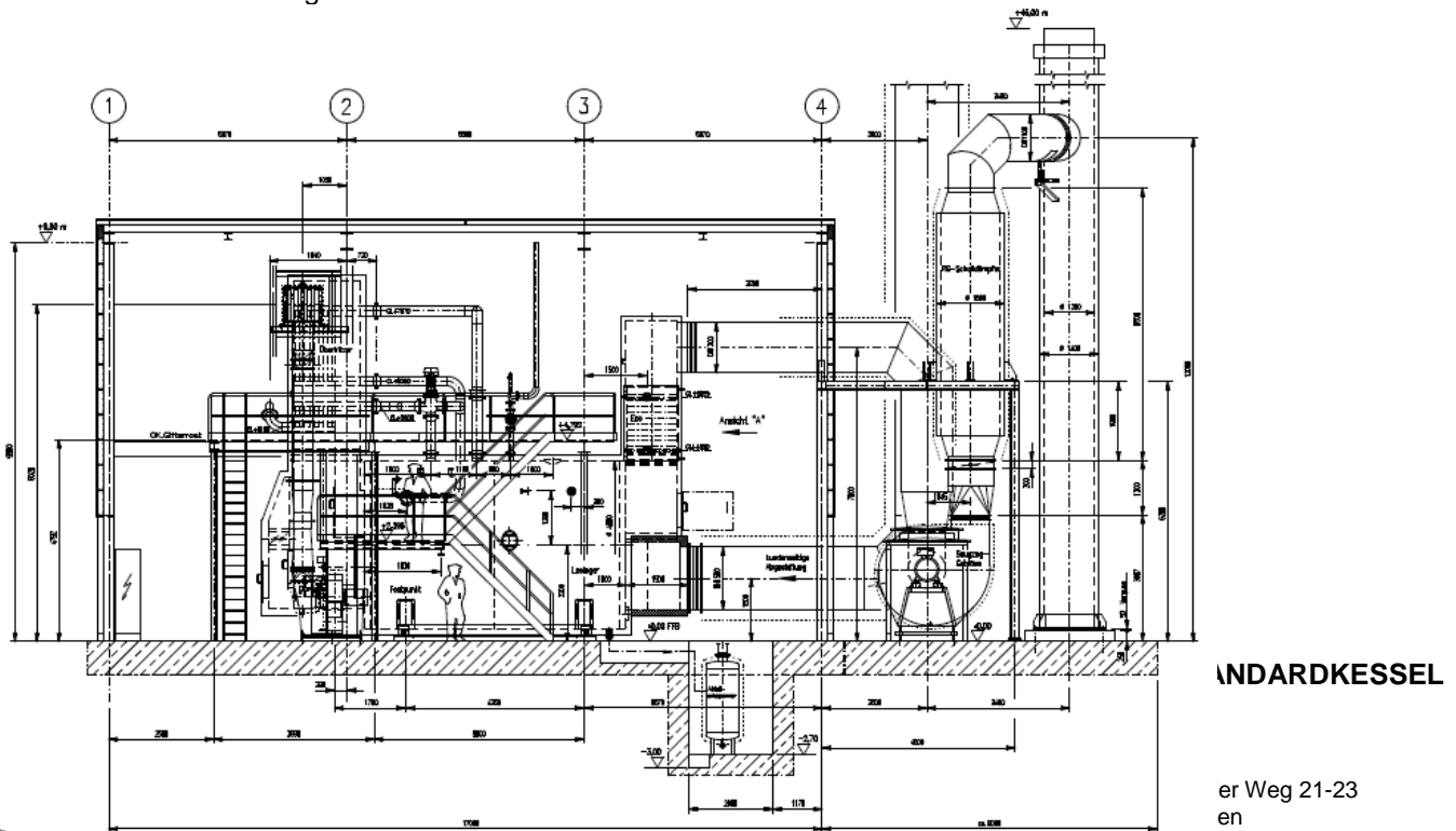
Bild 4 Kesselhaus mit Saugzugventilator, Schalldämpfer und Kamin.
