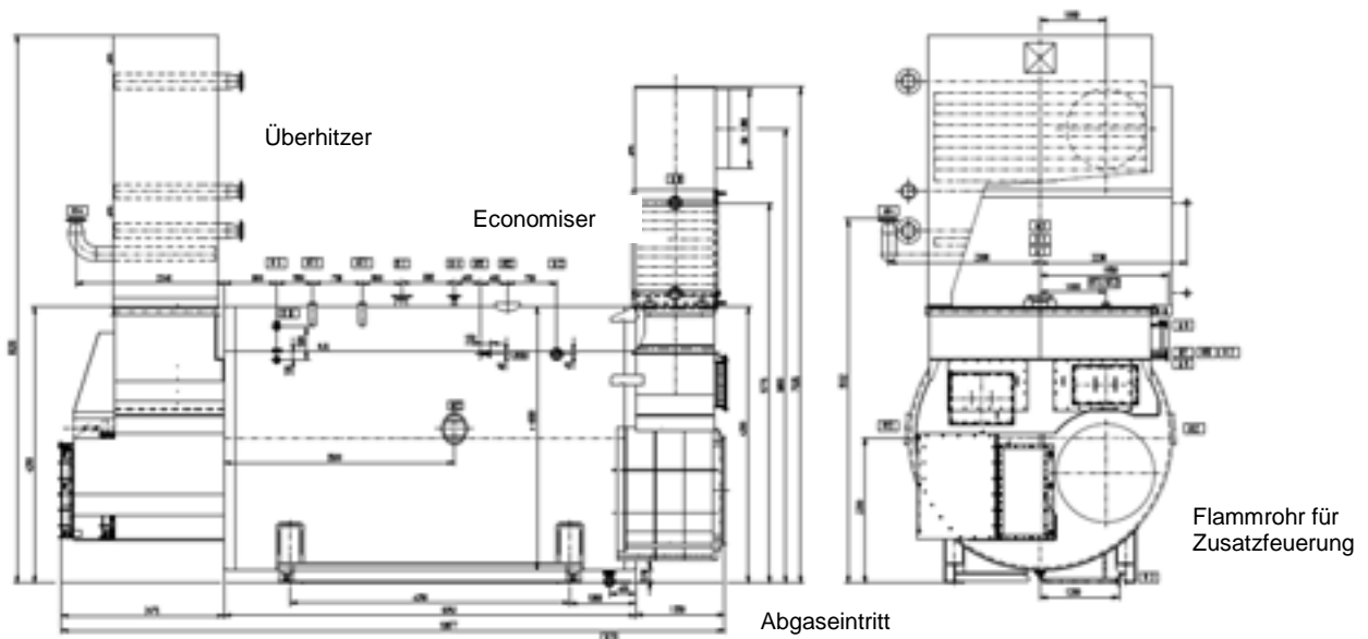
Bild 3 Kessel-Zusammenstellung
